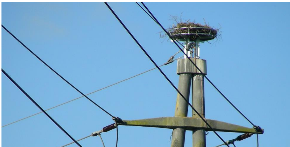
Horstunterlage mit Nistmaterial bietet Schutz vor Stromschlag.
